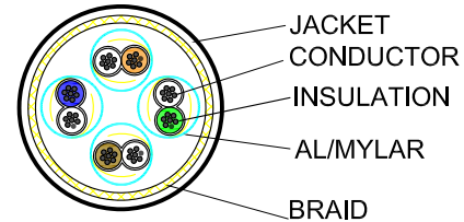
SEC:A-A
