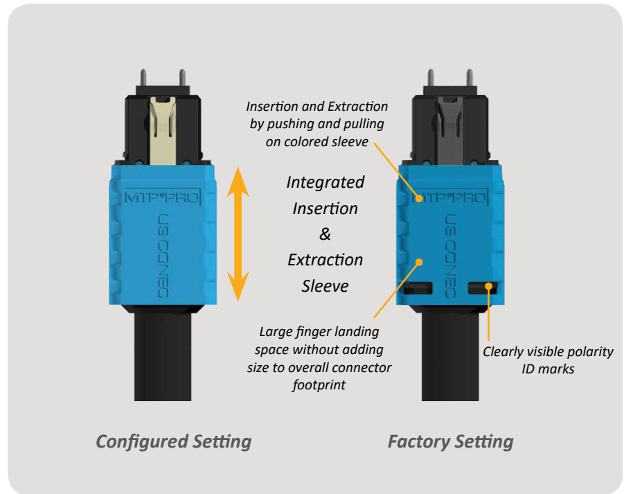
MTP® PRO
