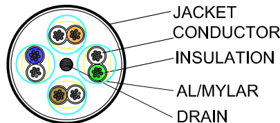
SEC:A-A
